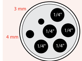
Mehrfachbohrung M05
