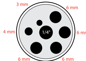
Mehrfachbohrung M02
