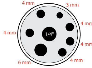
Mehrfachbohrung M01
