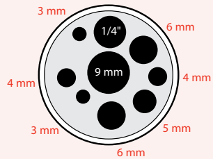
Mehrfachbohrung M04
