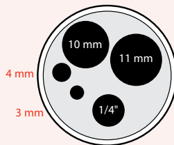
Mehrfachbohrung M09
