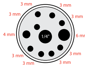
Mehrfachbohrung M03
