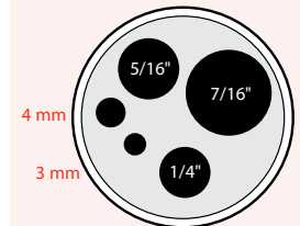
Mehrfachbohrung M10
